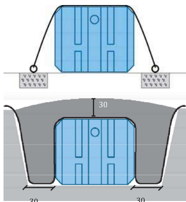
Esimerkki ankkuroinnista betoniin tai kalliioon.
